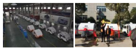
小水滴拖挂车生产流水线
